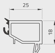
Spessore vetro 26-28mm Glass thickness 26-28mm
