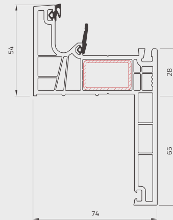
Telaio a ZETA 60 mm ZETA frame 60mm
