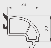
Arrotondato Rounded
